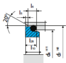
G6 (EN 12756)
